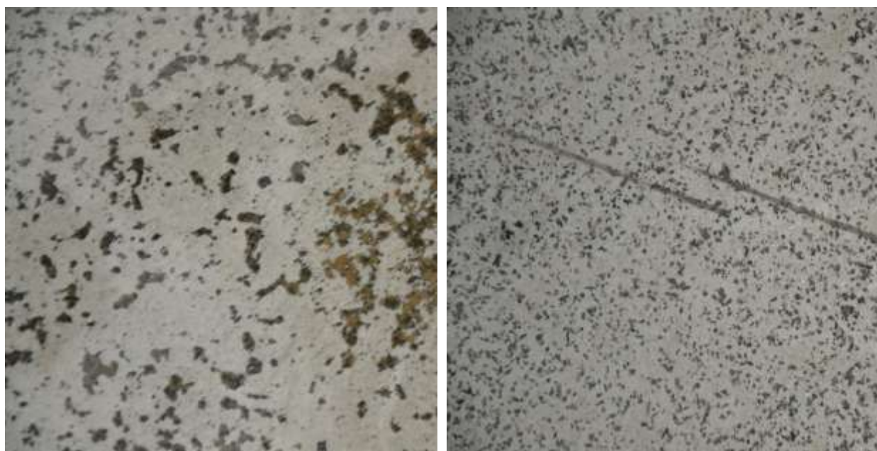
Figur 2.18 Slitage på Polyuretan Mapefloor PU efter 5 år på parkeringsdäcket i Kville
