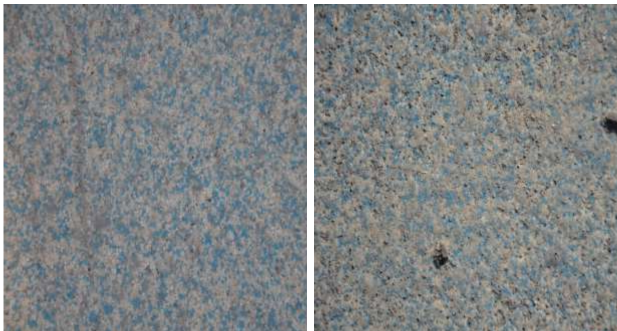
Figur 2.31 Akryl Silikal med mer än ytligt slitage efter dubbdäck samt gropar efter drygt 3 år på parkeringsdäcket i Baggen
