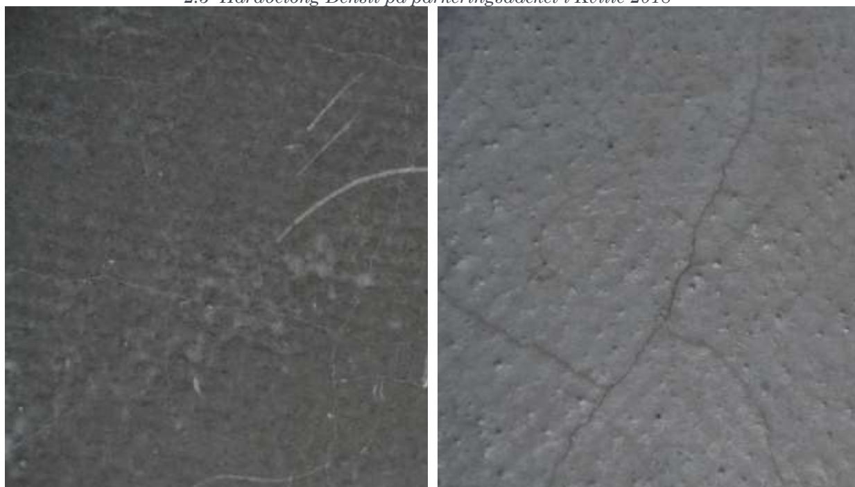
Figur 2.4 Ytligt slitage efter dubbdäck samt krackelering på hårdbetong Densit efter 5 år på parkeringsdäcket i Kville
